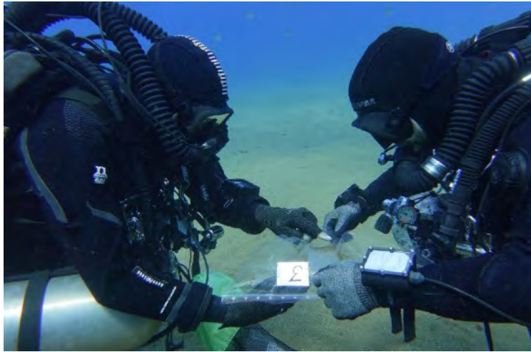
#8 Mise en place du système acoustique à effet Doppler pour la mesure du courant
